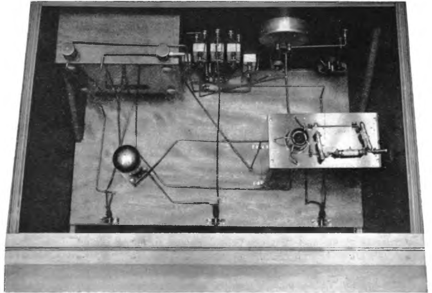
Fig. 4. Het beschreven instrument van binnen gezien. Rechts ziet men de opstelling van de voet van haar beroofde gelijkrichtlamp.
