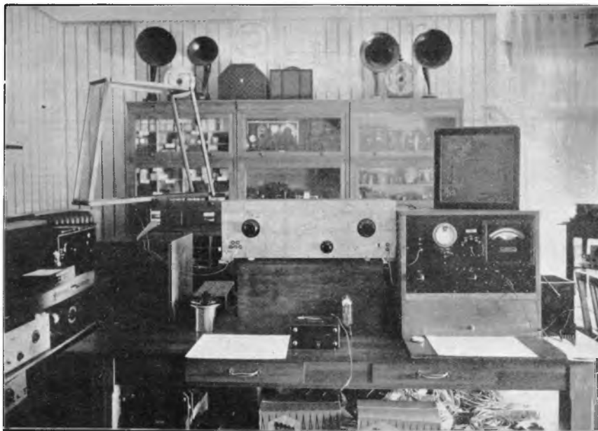
Fig. 9. De lampvoltmeter in gebruik op het laboratorium van den schrijver.
