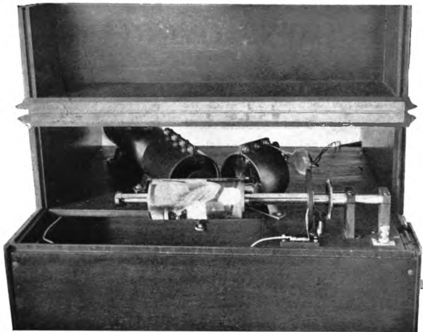
R.W.'s beeldzender van boven gezien. Links de „licht-richter”, daarnaast een lenzen-magazijn dat het door de foto gereflecteerde licht op de foto-cel werpt. Op den voorgrond de met een foto gespannen beeldwals, rechts daarvan de synchronisator
