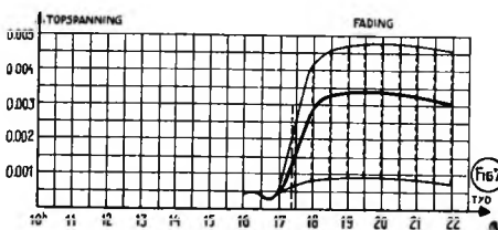
Hoogfreq. spanning van Praag (348.9 M) in raam-antenne.
